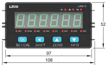
(正视图)
